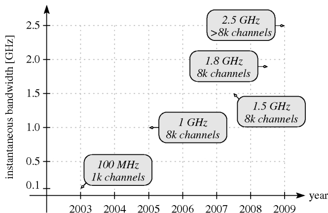
Fig. 1 FFTS developments at the Max-Planck-Institut für Radioastronomie.
